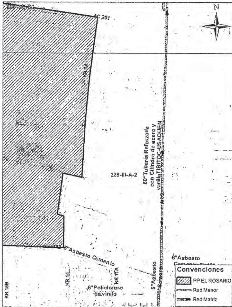
Ilustración 2. Redes de acueducto existentes – Desde la KR 15B a la AK 9 y entre la CL 192 y 1a AC 201.
