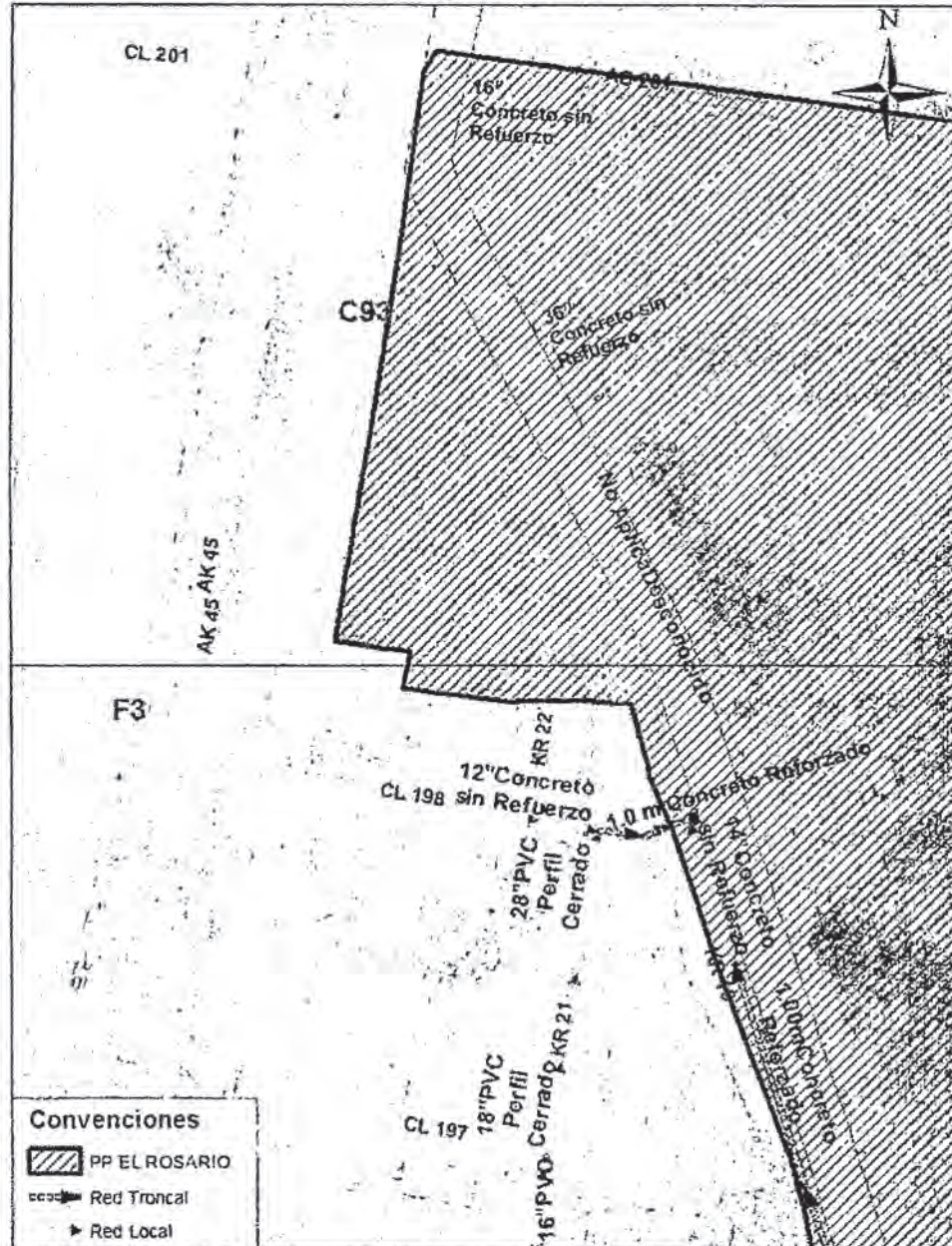
Ilustración 7. Redes de alcantarillado pluvial existentes – Desde la AK 45 a la KR 18 y entre la CL 197 y la CL 201.
