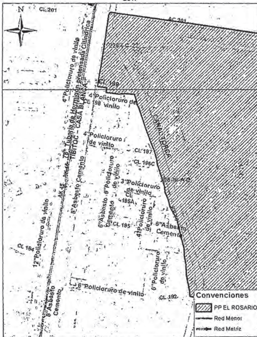
Ilustración 1. Redes de acueducto existentes – Desde la AK 45 a la KR 18 y entre la CL 192 y la CL 201.
