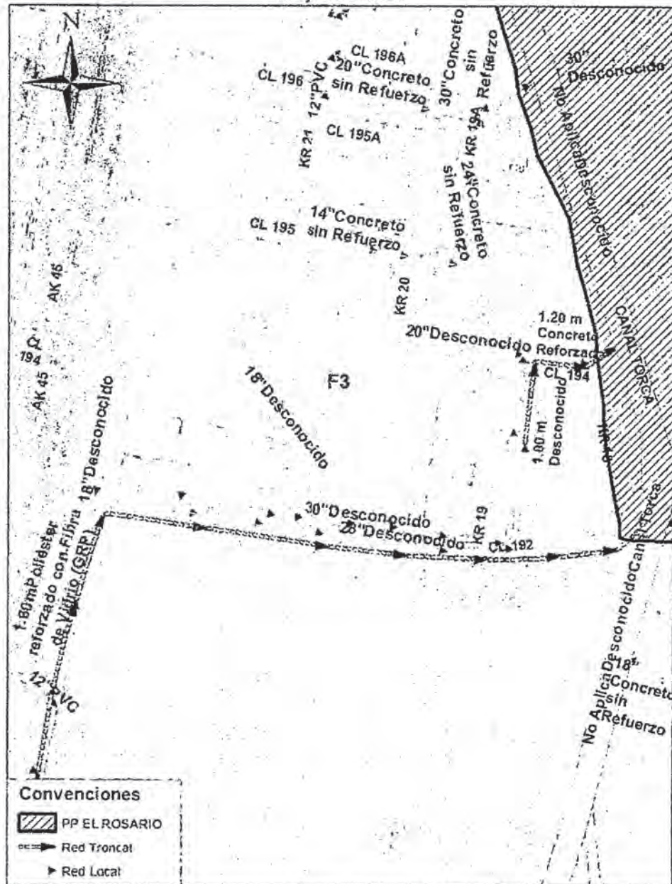
Ilustración 4. Redes de alcantarillado pluvial existentes – Desde la AK 45 a la KR 18 y entre la CL 192 y la CL 196A.
