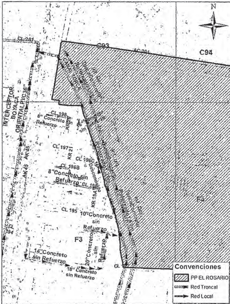
Ilustración 3. Redes de alcantarillado sanitario existentes – Desde la AK 45 a la KR 18 y entre la CL 192 y la CL 201.
