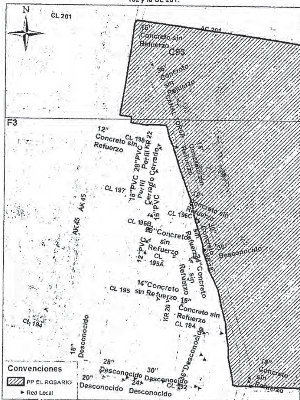
Ilustración 8. Redes de alcantarillado pluvial existentes – Desde la AK 45 a la KR 18 y entre la CL 192 y la CL 201.
