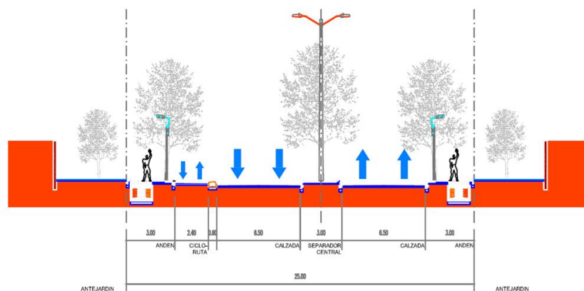
Imagen 8 Figura 1. Perfil vial I-4 Fuente: Decreto 555 de 2021
