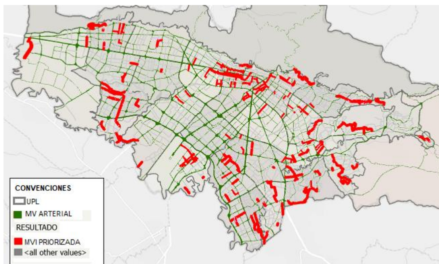
Imagen 169 Malla vial intermedia identificada por SDM. Fuente: SDM
