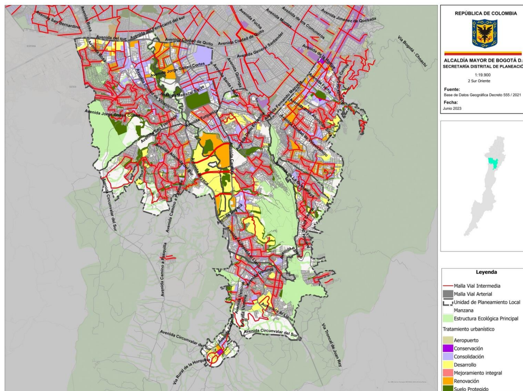
Imagen 187 Conectividad tratamientos urbanísticos mediante MVI propuesta- sector Suroriente
