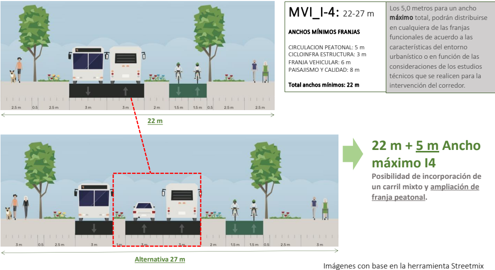
Imagen 95. Ejemplo perfiles franjas funcionales Fuente: DTS Definición de la Malla Vial Intermedia Sector Noroccidente – DPL, SDP
