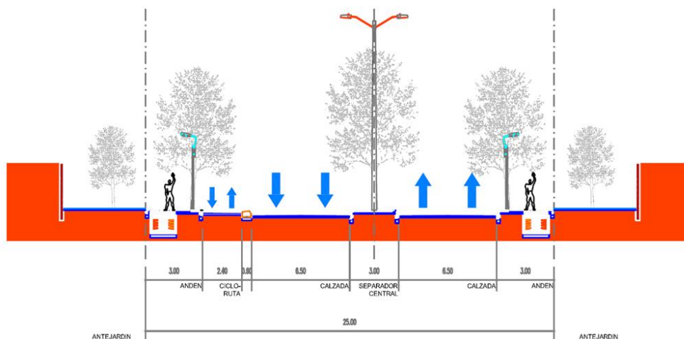
Imagen 90 Figura 1. Perfil vial I-4 Fuente: Decreto 555 de 2021
