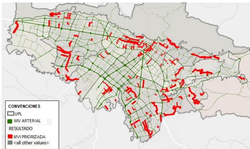
Imagen 104. Malla vial intermedia identificada por SDM Fuente: DTS Definición de la Malla Vial Intermedia Sector Noroccidente – DPL, SDP
