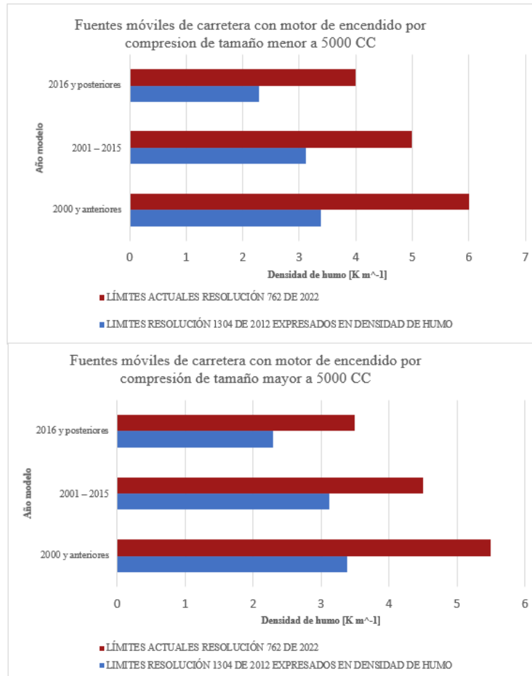
Figura 1 Comparativo de los límites de emisión de la Resolución 0762 de 2022 del Ministerio de Ambiente y Desarrollo Sostenible y la Resolución 1304 de 2012 de la SDA expresados en densidad de humo
