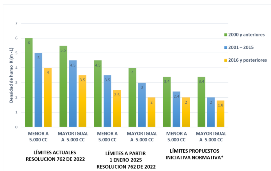
Figura 6 Comparativo de límites en Densidad de humo de acuerdo con lo establecido en la Resolución 762 de 2022
