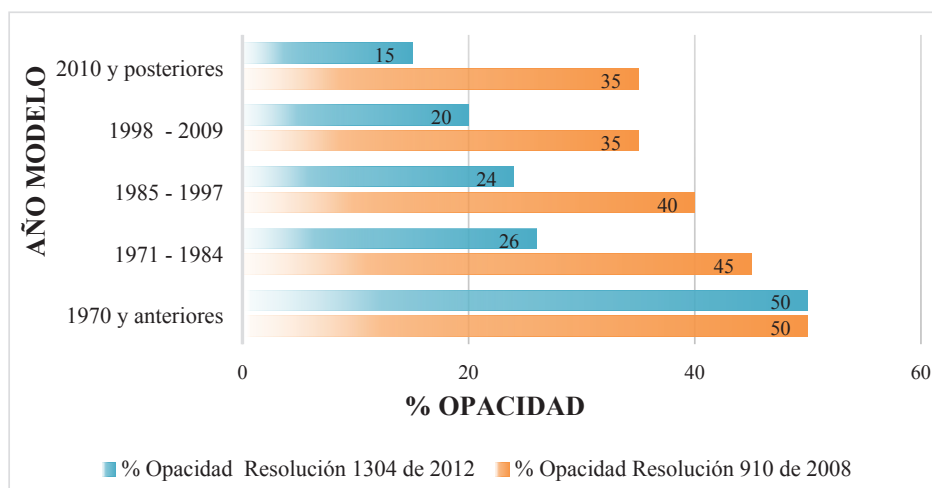
Figura 5 Comparativo de Límites entre Resolución 910 de 2008 y Resolución 1304 de 2012 para Opacidad
