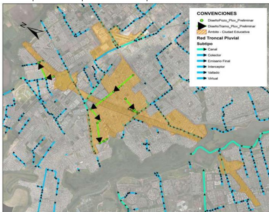
Ficha 63. Propuesta diseño conceptual redes alcantarillado pluvial
