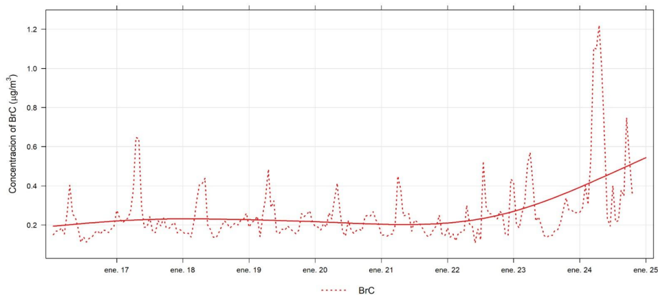
Figura 5. Serie temporal de BrC los últimos 8 días.
