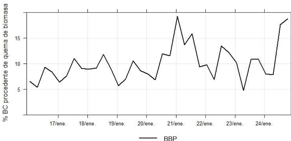
Figura 6. Serie temporal del porcentaje de eBC procedente de quema de biomasa.
