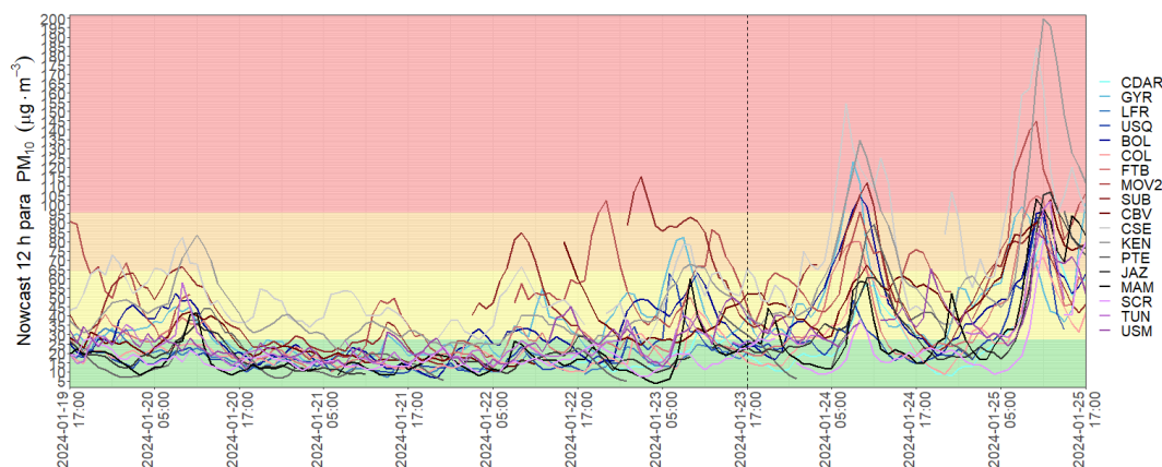
Figura 2. Comportamiento media móvil PM_{10} a nivel ciudad
