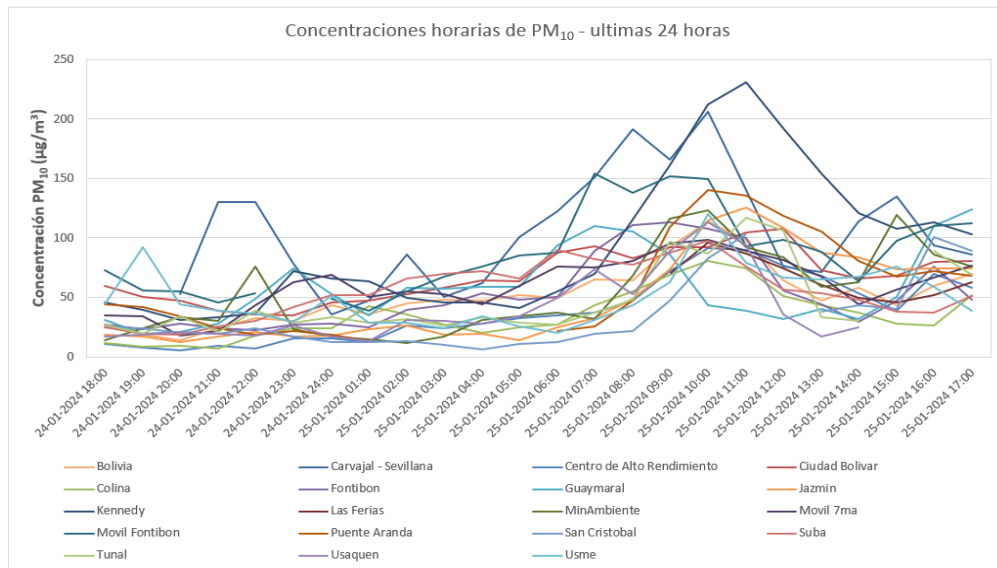
Figura 1. Concentraciones horarias para PM_{10} las últimas 24 horas.
