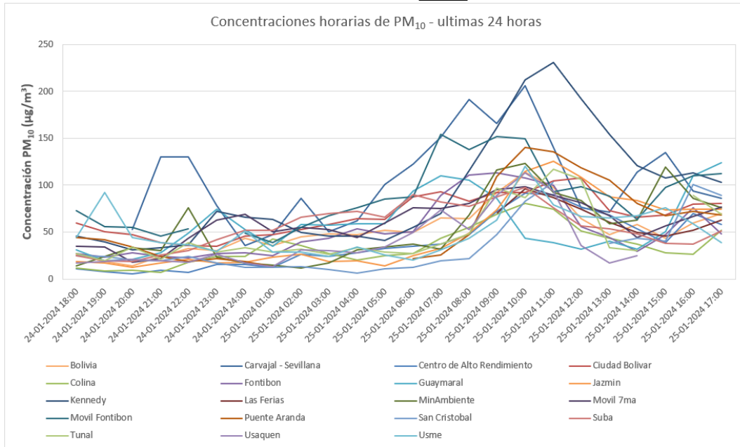
Figura 1. Concentraciones horarias para PM10 las últimas 24 horas.
