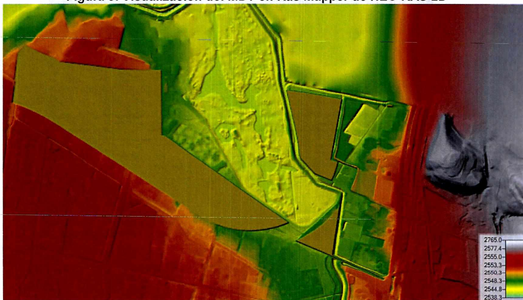
Figura 9. Visualización del MDT en Ras Mapper de HEC-RAS 2D
