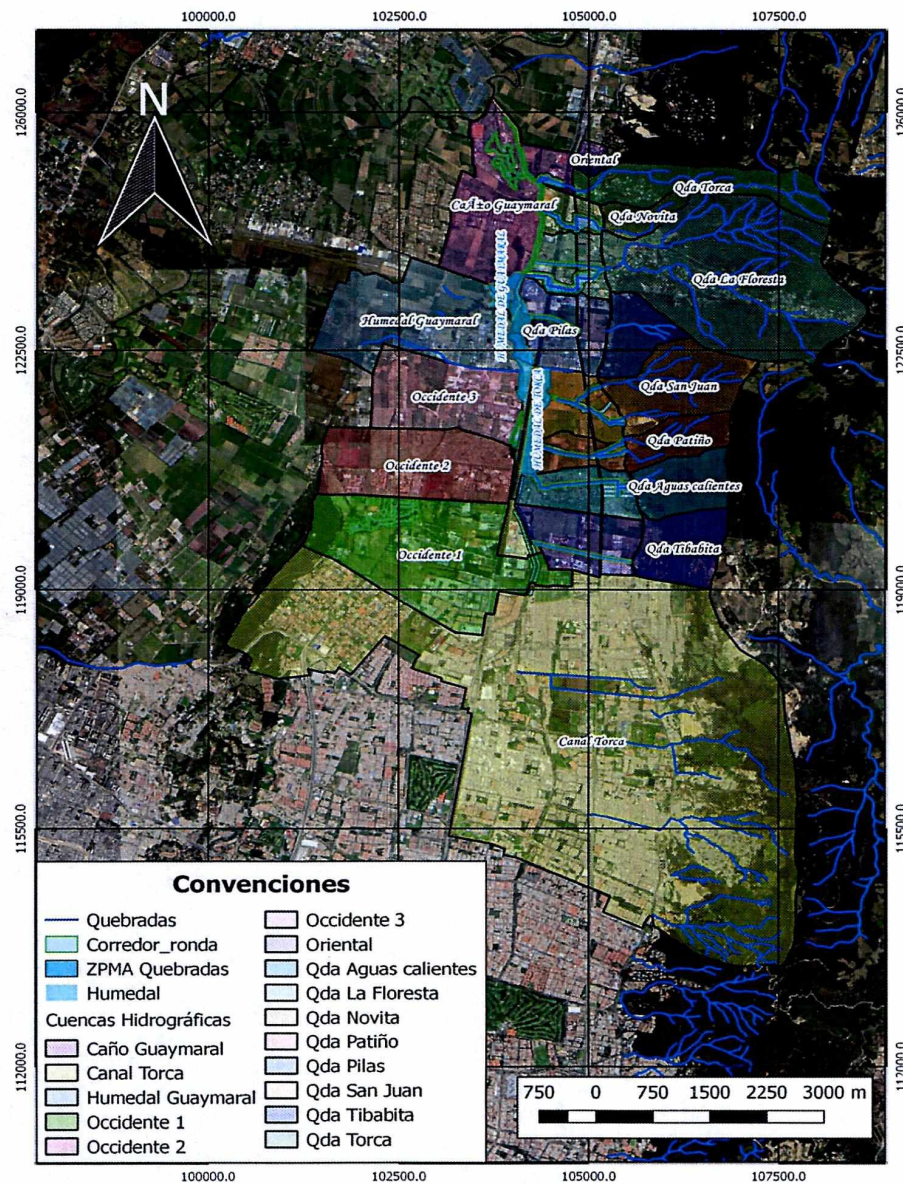
Figura 7. Detalle de áreas de aporte del sistema hídrico Torca-Guaymaral
