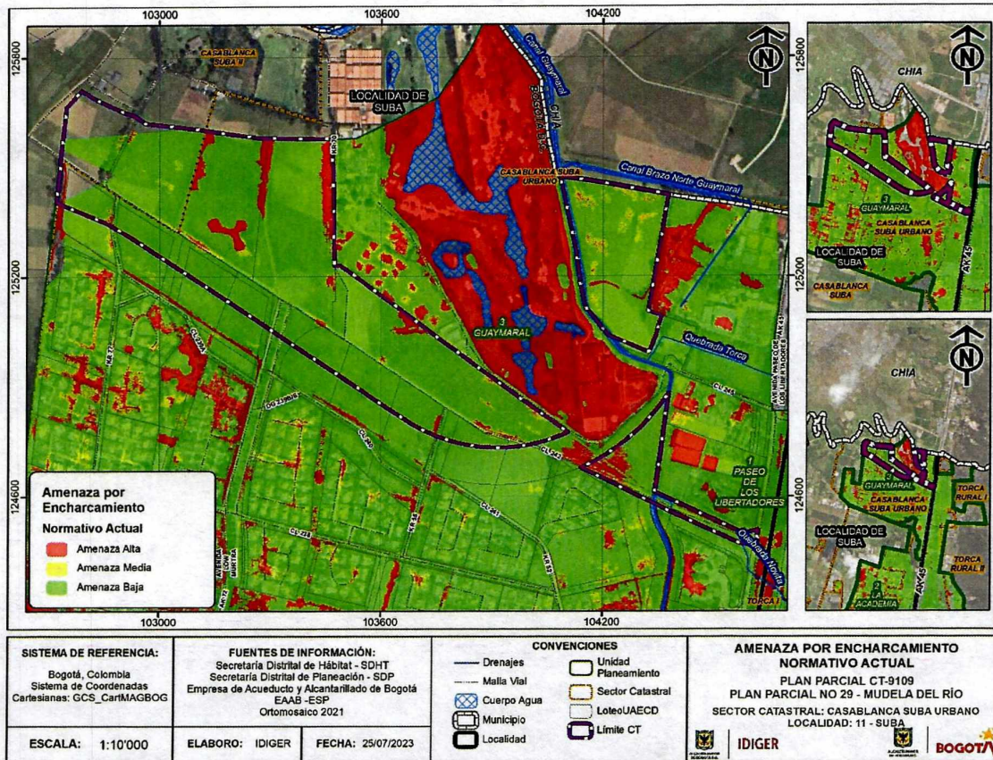
Figura 5. Condición de amenaza de inundación por encharcamiento (Decreto 555 DE 2021)
