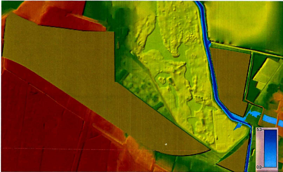
Figura 11. Extensión de la inundación periodo de retorno 100 años escenario prospectivo
