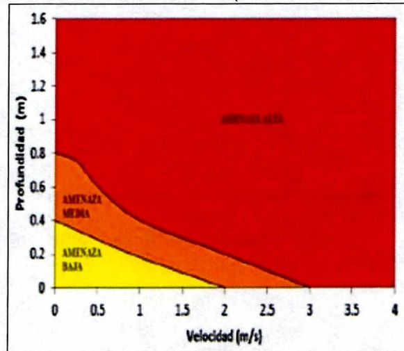
Figura 12- Evaluación de Amenaza (Extraída Estudios del IDEAM)
