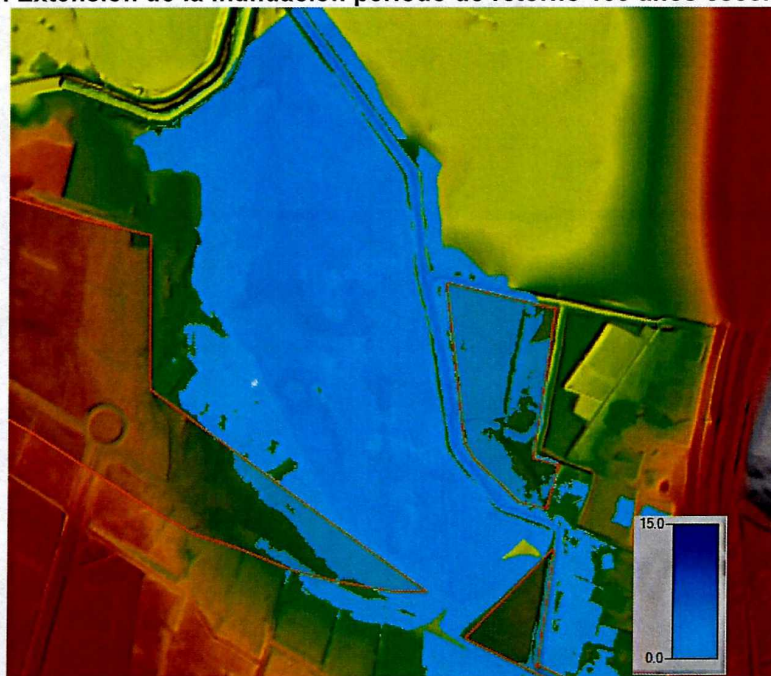
Figura 10. Extensión de la inundación periodo de retorno 100 años escenario actual
