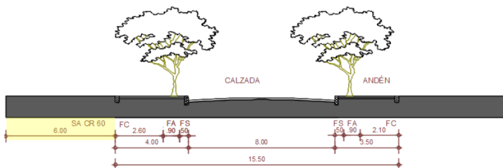
Figura 5. Secciones viales perimetrales con sobreanchos de andenes previstos por el PPRU Textilia
