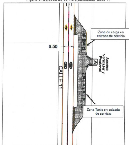
Figura 5. Calzada de servicio pacificada Calle 11
