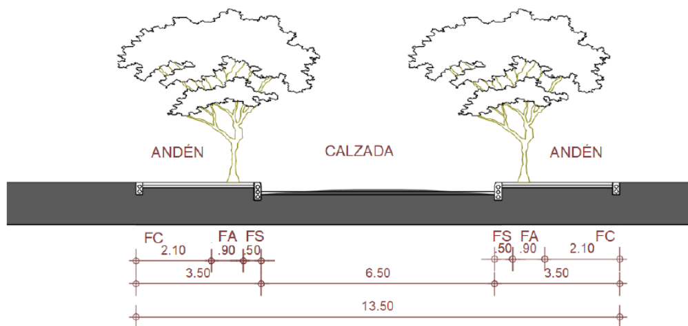
Figura 4. Reconfiguración de la sección vial Calle 11 y Calle 12
