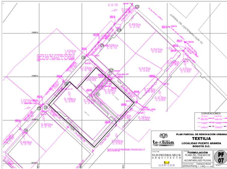
Imagen Plano 23. Plano PF-07 Trazado de Redes de Alcantarillado Pluvial Fuente: Consultoría Hidráulica y Urbanismo LTDA.
