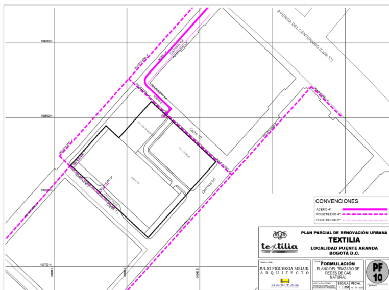
Imagen Plano 26. Plano PF-10 Trazado de Redes de Gas Natural Fuente: Consultoría Gas Natural VANTI -JFM.
