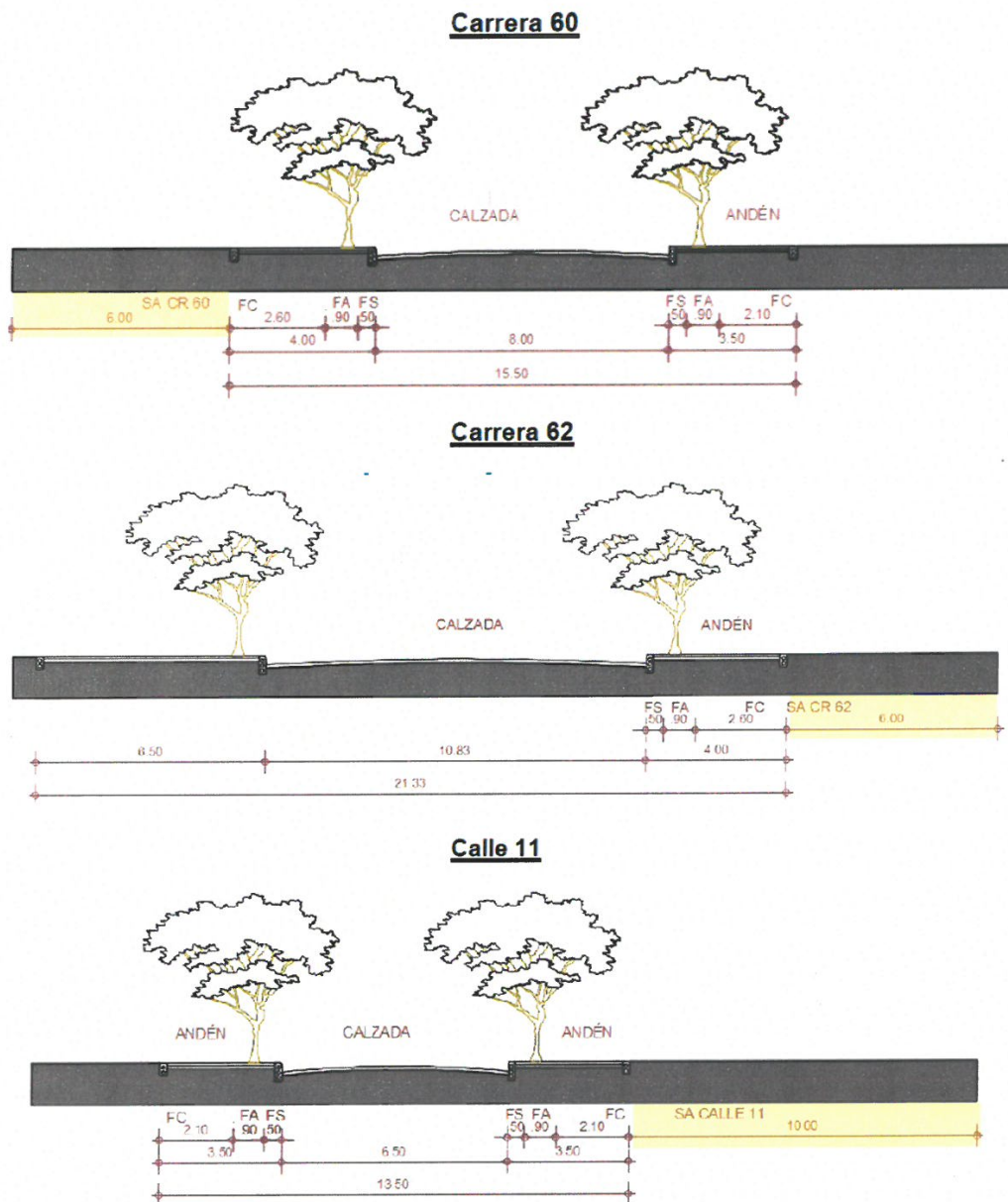
Figura 3. Secciones viales perimetrales con sobreanchos de andenes previstos por el PPRU Textilía
