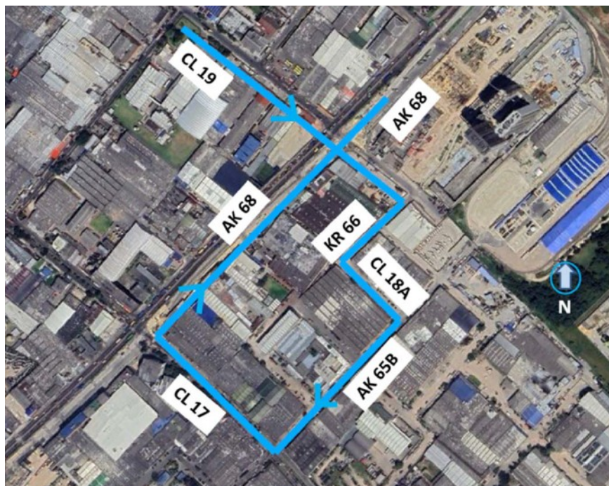
Figura 2. Trayectorias de desvío camiones C4 y superior
