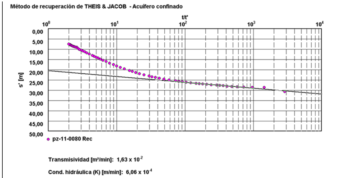
Figura 1. Curvas de interpretación de la prueba de bombeo a partir de los datos de bombeo y recuperación en el pozo pz-11-0080
